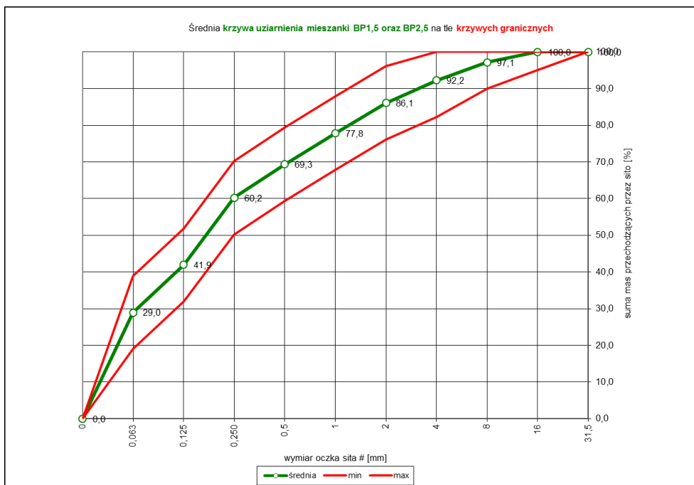
Rysunek 1 Krzywe graniczne mieszanki betonowej BP 1,5 oraz BP 2,5
